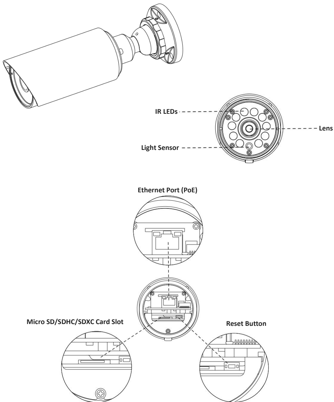
Figure 1-3-5 Mini Bullet Network Camera
