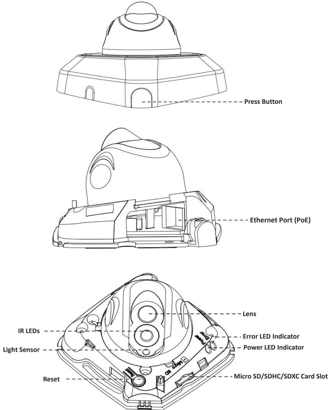
Figure 1-3-2 IR Mini Dome Network Camera
